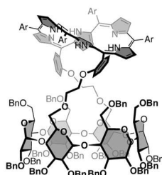
[28]10 (Ar = C 6 F 5 )
