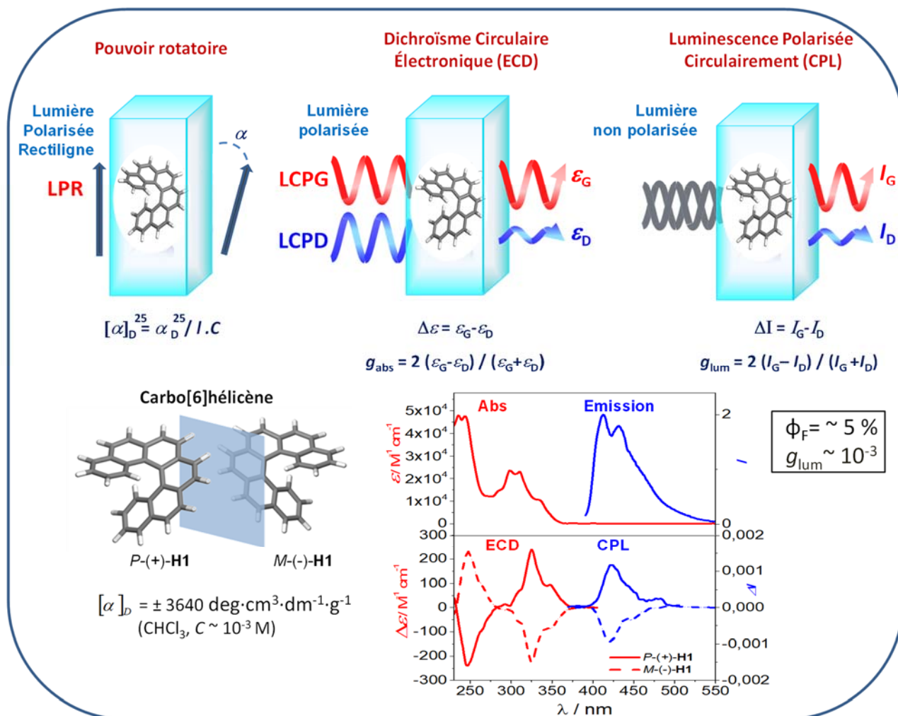
Figure 1: les énantiomères P et M du carbo[6]hélécène (noté H1 ). Principes du pouvoir rotatoire, du dichroïsme circulaire électronique et de l'émission polarisée circulairement. \alpha est l'angle de rotation de la lumière polarisée rectilignement (voir les définitions). g_{abs} et g_{lum} sont appelés facteurs de dissymétrie, respectivement en absorption et en émission. \epsilon_D et \epsilon_G (resp. I_D et I_G ) sont respectivement les coefficients d'extinction molaire (resp. intensités émises) pour une lumière polarisée circulairement droite et gauche [3].
