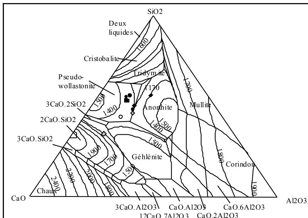
Figure 3 : Localisation des analyses chimiques des verres du CEA CAD (carrés noirs), des vitriats de REFIOM vitreux (losanges noirs), des vitriats de REFIOM cristallisés (losanges blancs), des scories paléosidérurgiques de Rogéville et de Sexey-aux-Forges (ronds noirs) et de Frouard (rond blanc), dans le diagramme \text{SiO}_2 - \text{CaO} - \text{Al}_2\text{O}_3
