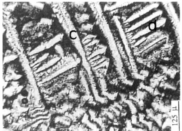
Photo 2 : Vitrifiat « cristallisé » : assemblage de cristaux de méllilites (c) et sphènes (d) dans une matrice vitreuse
