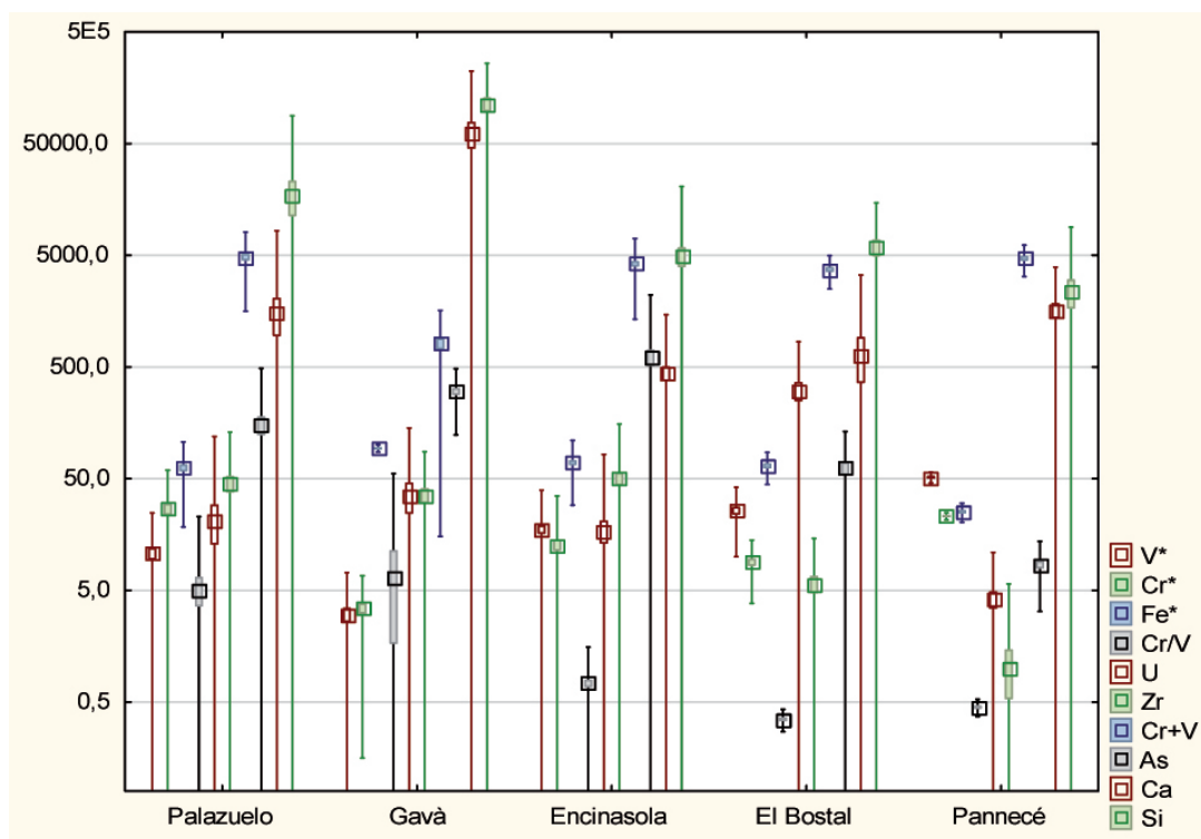
Fig. 3 : Comparaison des cinq gisements européens de variscite sur la base des variations prises en compte dans le modèle chimio-métrique : V*, Cr*, Fe* (valeurs normalisées à 100% par rapport à V+Cr+Fe), le rapport Cr/V, les concentrations en U, Zr, (Cr+V), As, Ca et Si.
