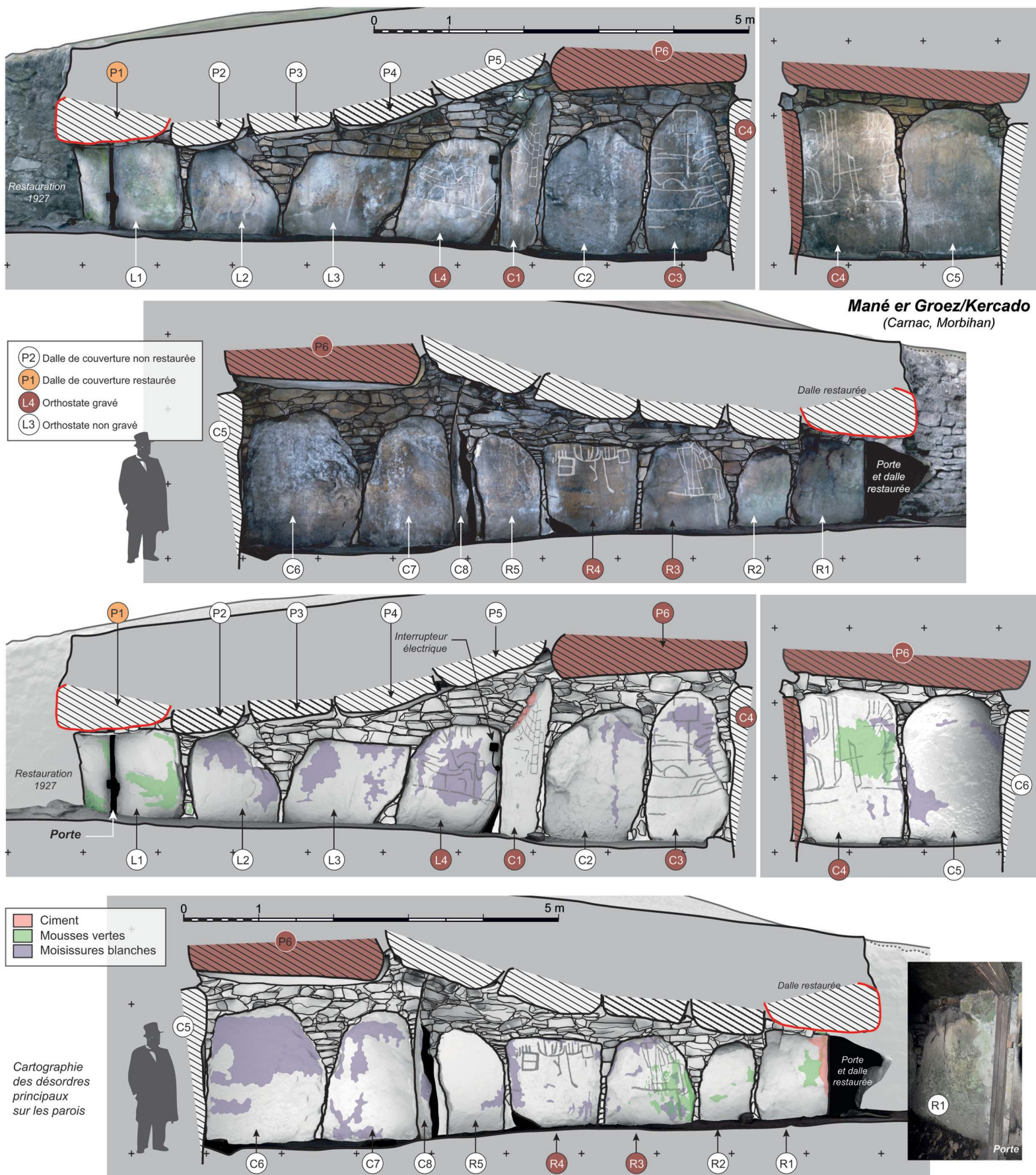
Fig. 4 – Élévations de la tombe à couloir du Mané er Groez : orthophotographies mosaïques et inventaire des principaux désordres sur le modèle photogrammétrique (occlusion ambiante ; DAO S. Cassen, modèle 3D V. Grimaud et H. Paitier).
