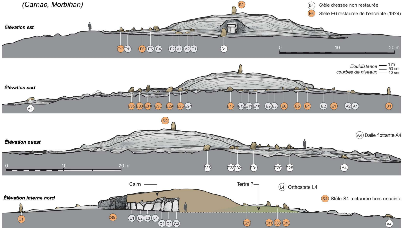
Fig. 2 – Site de Kercado (Carnac). Élévations du cairn du Mané er Groez et de l’enceinte de stèles, et détection d’une anomalie de relief. Microtopographie sur modèle en occlusion ambiante (DAO S. Cassen, modèle 3D V. Grimaud). Site of Kercado (Carnac). Elevations of the cairn of Mané er Groez and the standing stone enclosure; detection of a topographic anomaly. Microtopography on model in ambient occlusion (CAD S. Cassen, 3D model V. Grimaud).
