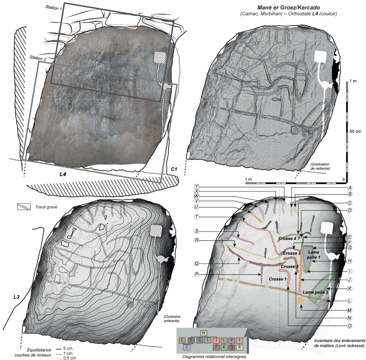
Fig. 15 – Orthostate L4 (couloir) : orthophoto mosaïque avec emplacements des fenêtres d’acquisition ICEO, microtopographie et levé redressé des gravures dans le modèle photogrammétrique (DAO S. Cassen, modèle 3D V. Grimaud). Orthostat L4 (passage): mosaic orthophoto with location of the ICEO acquisition windows, microtopography and rectified survey of the engravings in the photogrammetric model (CAD S. Cassen, 3D model V. Grimaud).
