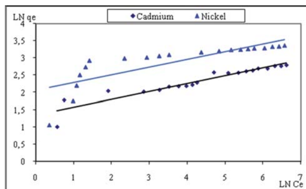
Fig. 19. Freundlich isotherm of the mixture \text{Ni}^{2+} and \text{Cd}^{2+} .
