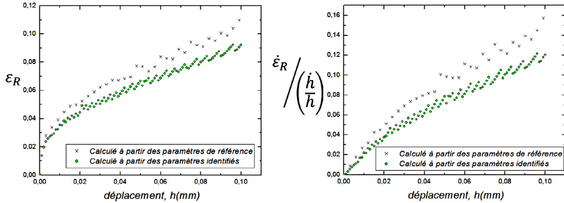
Fig. 5. (a) Déformation représentative et (b) vitesse de déformation représentative en fonction de la profondeur d'indentation obtenue à partir des jeux de paramètre de référence et les paramètres identifiés donnés dans le Tableau 1.
