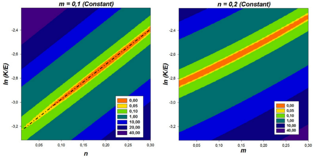
Fig. 2. Variation de la fonction objective Q_1 : (a) m = 0,1 , (b) n = 0,2 obtenue par simulation numérique d'un essai d'indentation sphérique avec une vitesse de pénétration \dot{h} = 1000 \mu\text{m.s}^{-1} .
