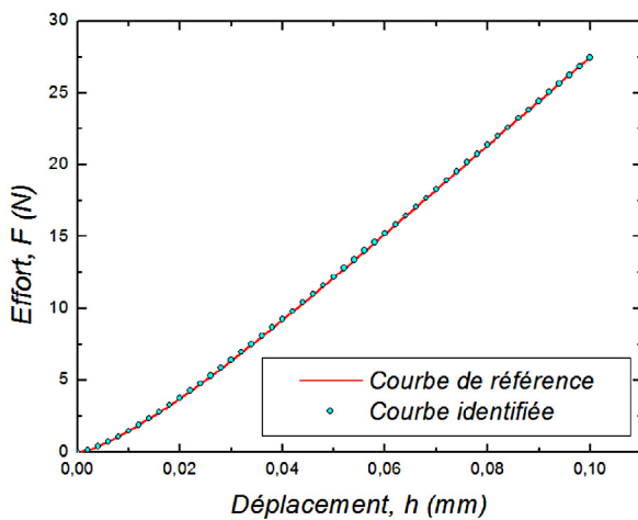
Fig. 4. Comparaison entre la courbe d'indentation de référence et la courbe obtenue par simulation numérique à partir du jeu de paramètre identifié présenté dans le Tableau 2.
