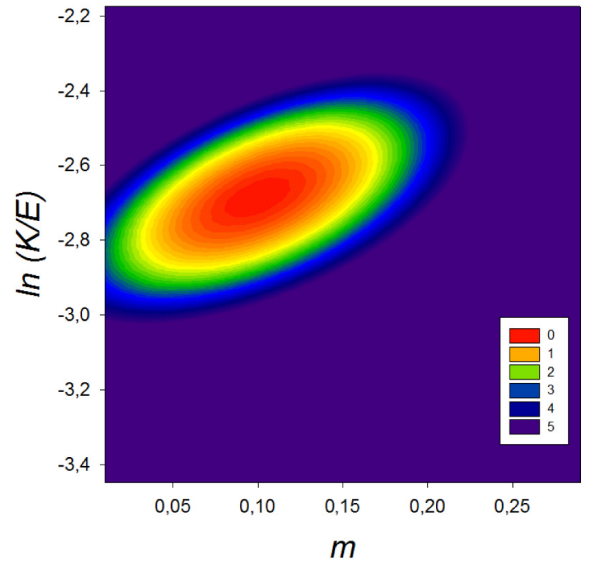
Fig. 3. Variation de la fonction objective Q_2 pour une valeur de n fixé à 0,2 obtenue à partir de 2 simulations d'indentation sphérique avec des vitesses de pénétration respectivement égales à h_1 = 10 \mu\text{m.s}^{-1} et h_2 = 1000 \mu\text{m.s}^{-1} .
