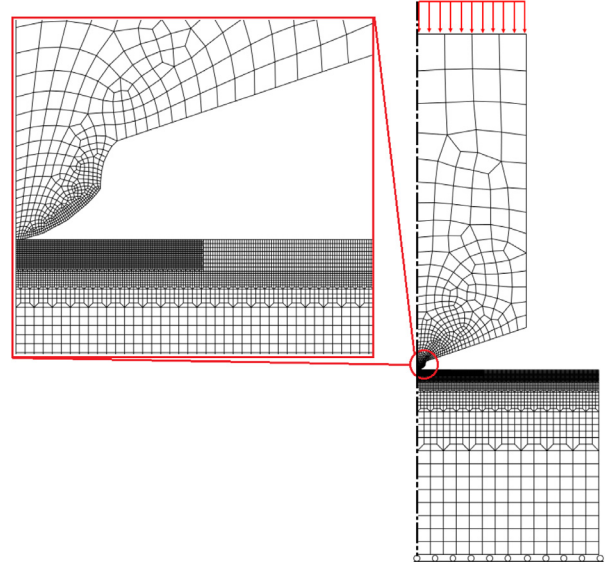
Fig. 1. Maillage utilisé pour la simulation numérique d'un essai d'indentation sphérique (Rayon de l'indenteur r = 0,25 \text{ mm} ).
